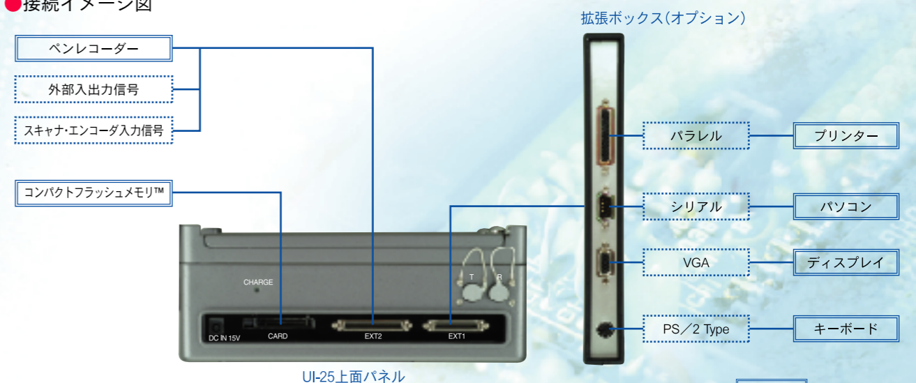
UI-25上面パネル
