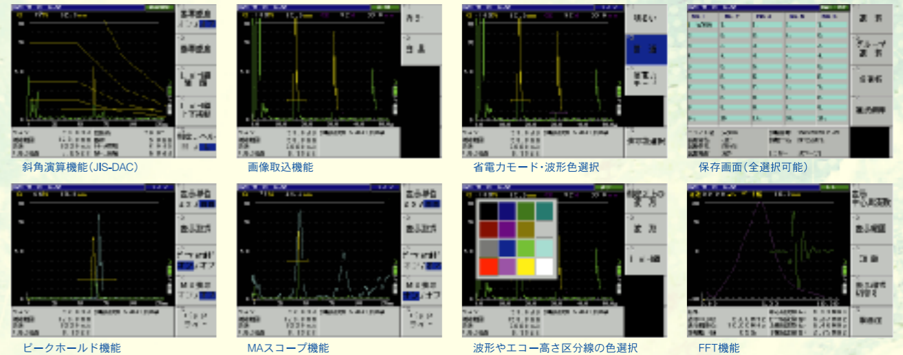
新JIS-DACによるRB-41試験片にて作成
